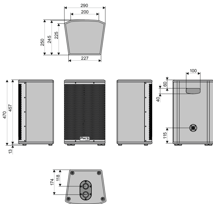
ГРОМКОГОВОРИТЕЛЬ-САТЕЛЛИТ DELTA3210
