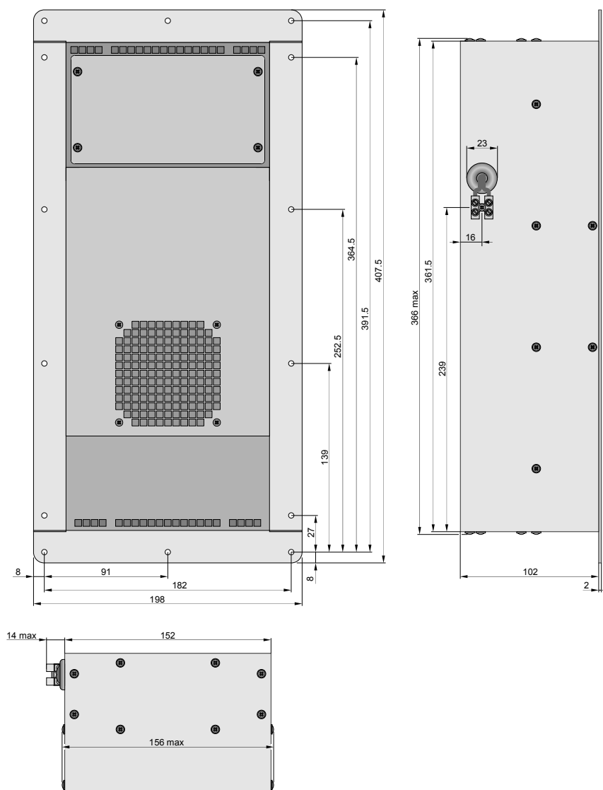
ГАБАРИТНЫЙ ЧЕРТЕЖ
