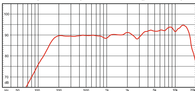
АЧХ громкоговорителя VA401i (processed)
