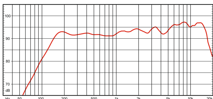
АЧХ громкоговорителя VA402i (processed)
