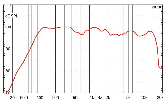
АЧХ монитора SM155
