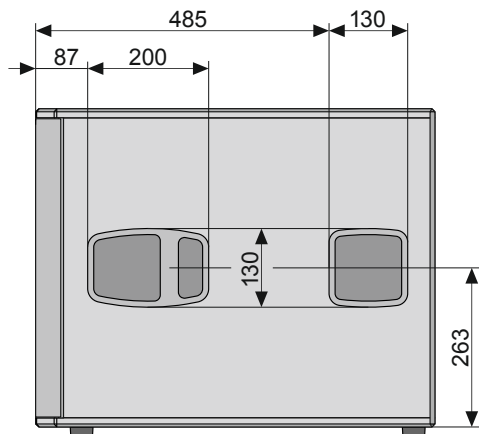
Side view / Вид сбоку (right / справа)
