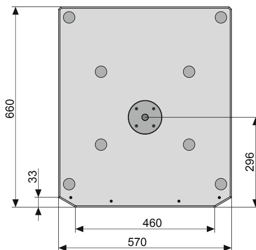
Top view / Вид сверху
