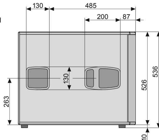
Side view / Вид сбоку (left / слева)
