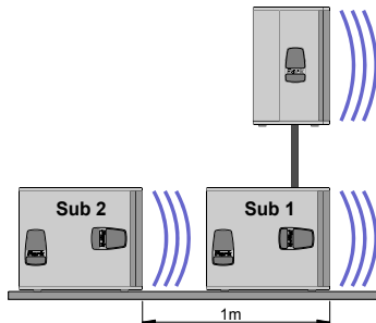
Градиентный массив
