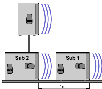
Массив «End-fire»
