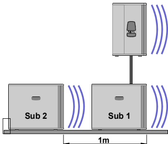
Градиентный массив
