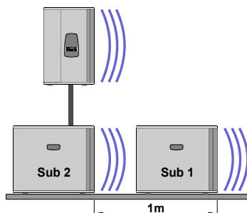
Массив «End-fire»
